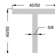
▲ Paletti ▼ Sezione
