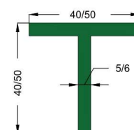
▲ Paletti ▼ Sezione
